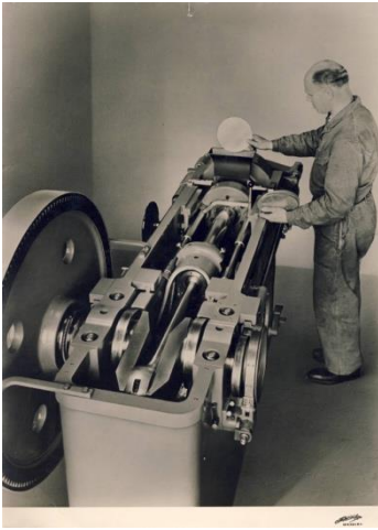
Hans Gloor an der Tiefziehpresse für Konservendosen
